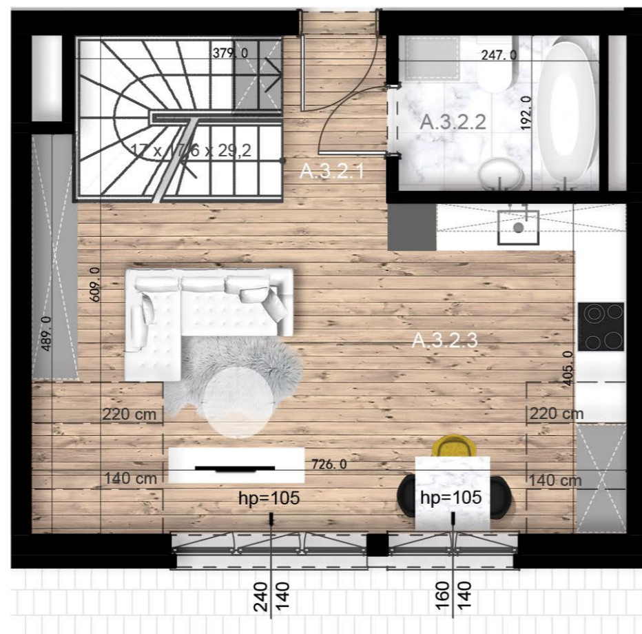
Poziom +3
